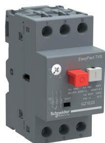
GZ1 E
